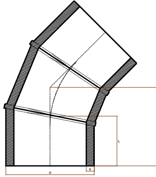
KONFEKSİYON 45 ° DİRSEK SEGMENTED 45 ° ELBOW COUDE SEGMENTÉ 45° / ОТВОД (Сварной) 45° / 45° (ملففة) كوع PE100 - SDR 17 - PN10 ve SDR 11 - PN16
