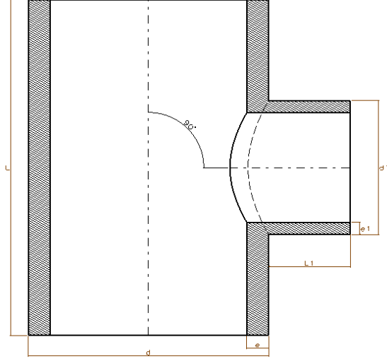
KONFEKSİYON İNEĞAL TE SEGMENTED REDUCED TEE PE100 - SDR 17 - PN10 ve SDR 11 - PN16
