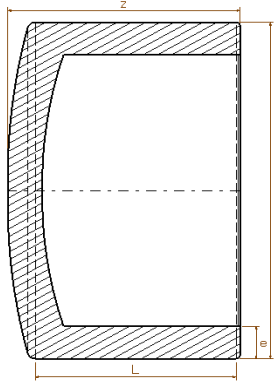
ENJEKSİYON KEP (KÖR TAPA) INJECTION CAP PE100 - SDR 17 - PN10 ve SDR 11 - PN16
