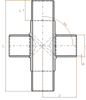
KİT ENJEKSİYON KAYNAKLI DÖRT KÖŞE TE KIT INJECTION WELDED CROSS TEE PE100 - SDR 17 - PN10 ve SDR 11 - PN16
