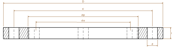
ÇELİK KÖR FLANŞ PN 10 STEEL BLIND FLANGE PN 10
